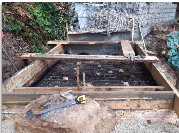
Coffrage de la 2 e partie de la dalle de répartition
